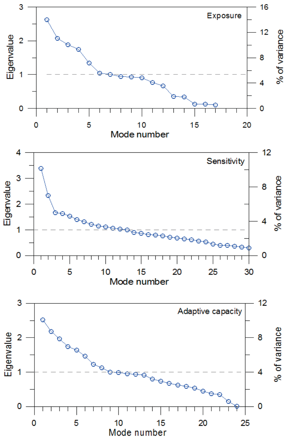
รูปที่ 4.36 ค่า eigenvalue และสัดส่วนความแปรปรวนในแต่ละโหมดของ PCA สำหรับองค์ประกอบหลัก Exposure, Sensitivity และ Adaptive capacity ของจังหวัดนครศรีธรรมราช
