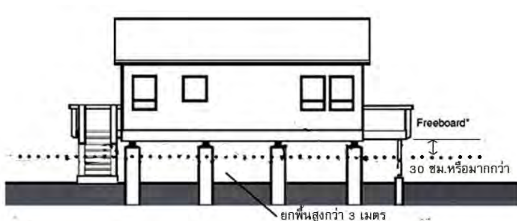
รูปที่ 7.27 แนวทางการกำหนดมาตรการด้านการออกแบบอาคารในพื้นที่เสี่ยงน้ำท่วมสูง
